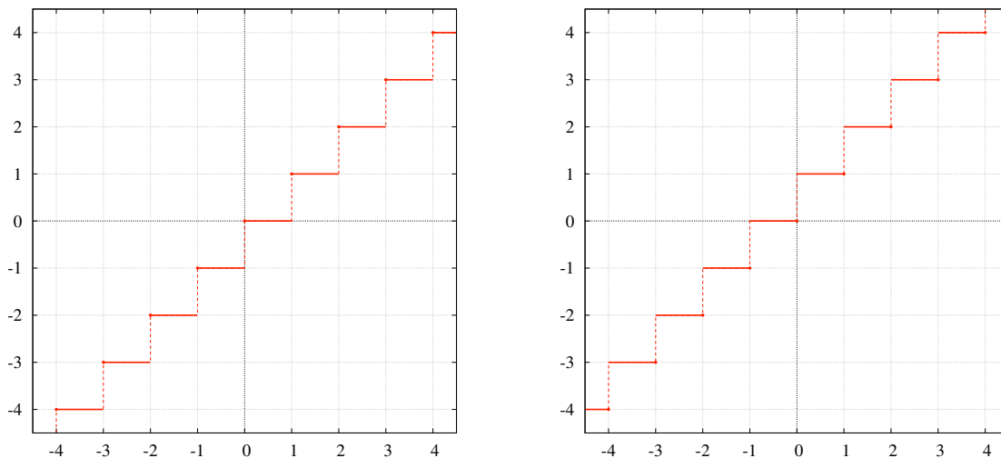
Figura 8.1: Gráficos da função piso \lfloor x \rfloor (à esquerda) e da função teto \lceil x \rceil (à direita).
