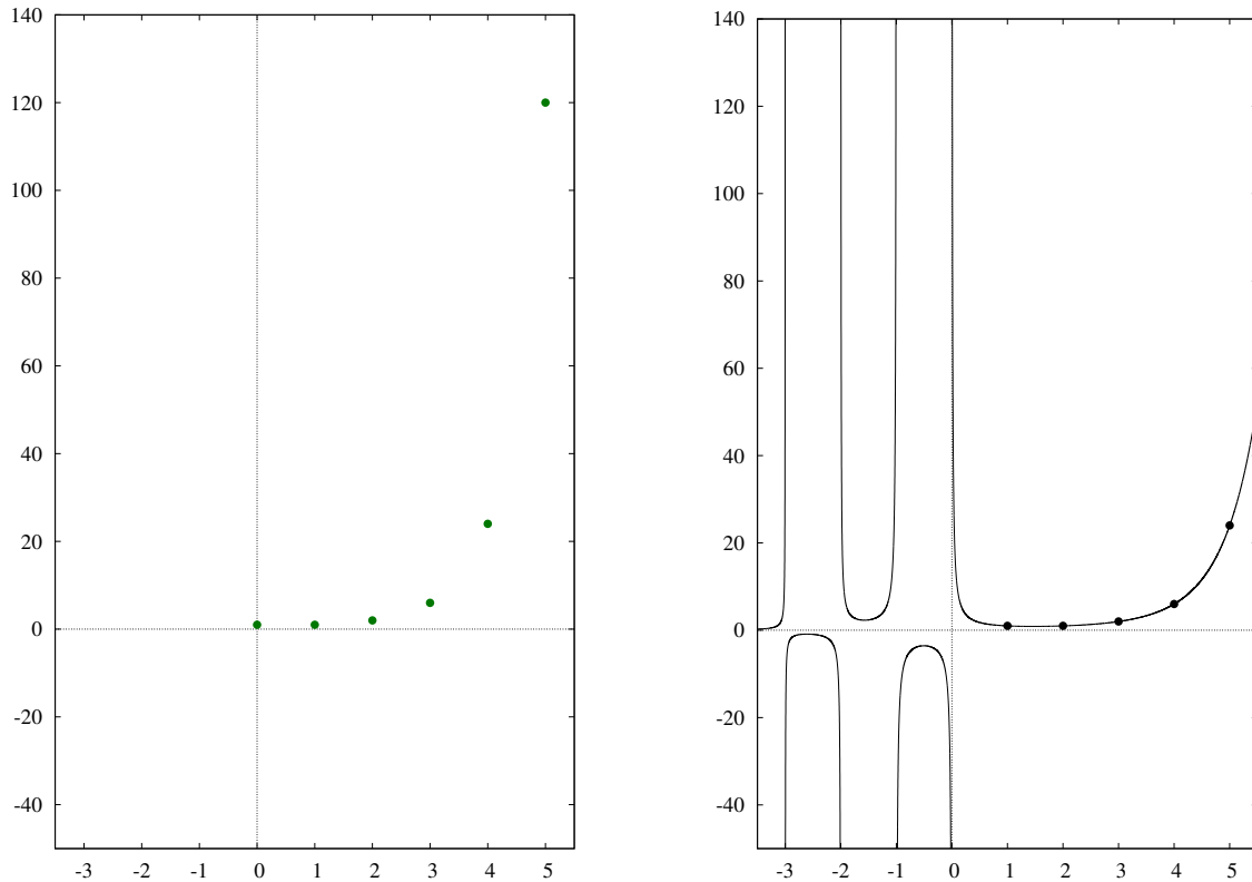
Figura 8.3: À esquerda, um gráfico da função fatorial, que dado n devolve n! , para n \in \{0, 1, \dots, 5\} . À direita, um gráfico da função \Gamma (linha contínua) e de (n-1)! (pontos).
