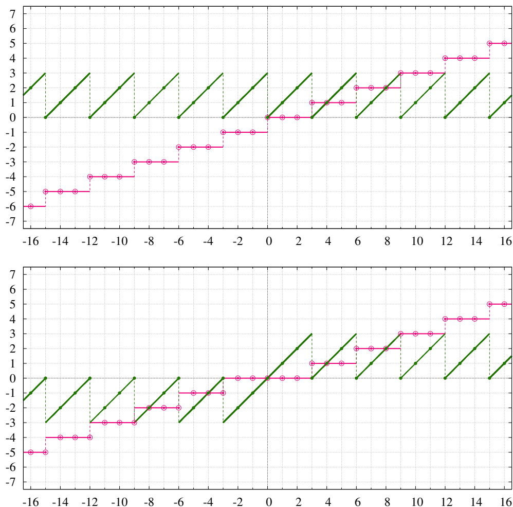
Figura 8.2: No alto, gráficos da função x \div 3 (vermelho) e x \bmod 3 (verde) para valores inteiros de x (pontos) e valores reais (linha). Em baixo, gráfico das operações análogas nas linguagens de programação C e Fortran.
